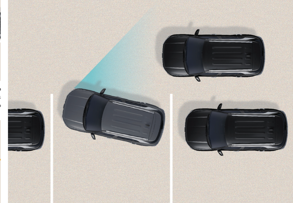
نظام مساعدة تجنب التصادم في النقاط العمياء (BCA) يُحذرك نظام مساعدة تجنب التصادم في النقطة العمياء (BCA) في حال وجود خطر اصطدام بمركبة خلفية في النقطة العمياء أثناء تغيير المسارات. عند الخروج من موقف مواز، وفي حال وجود خطر تصادم بمركبة تقترب من الخلف، يُساعدك النظام تلقائيًا في الفرملة الطارئة.
